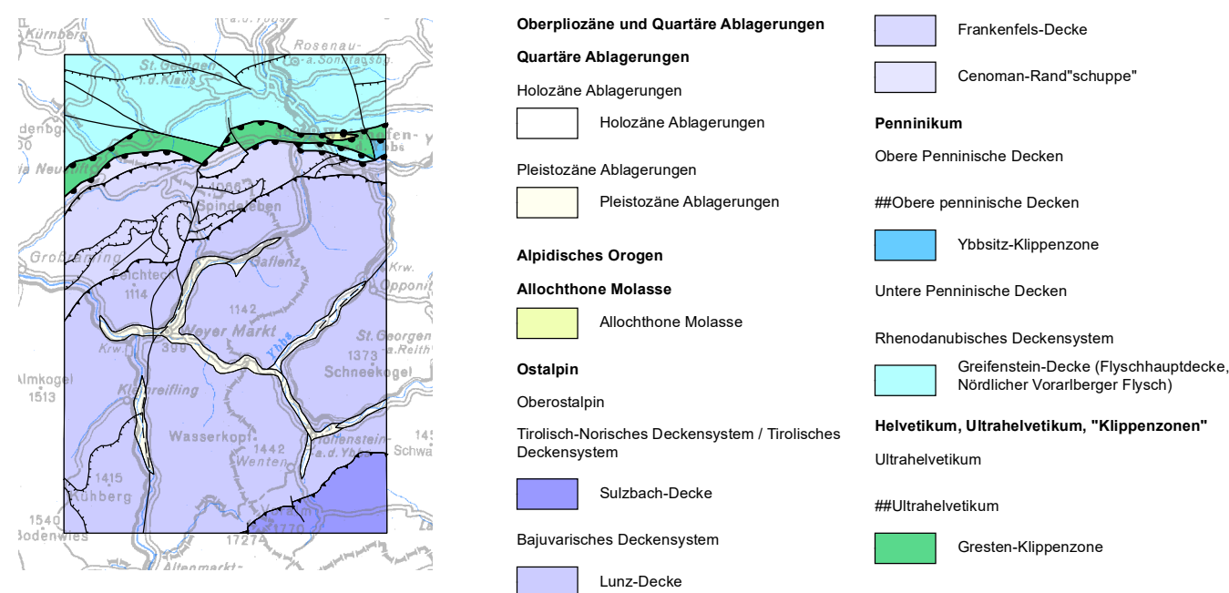
Geologisch-tektonische Übersicht 1: 400 000
